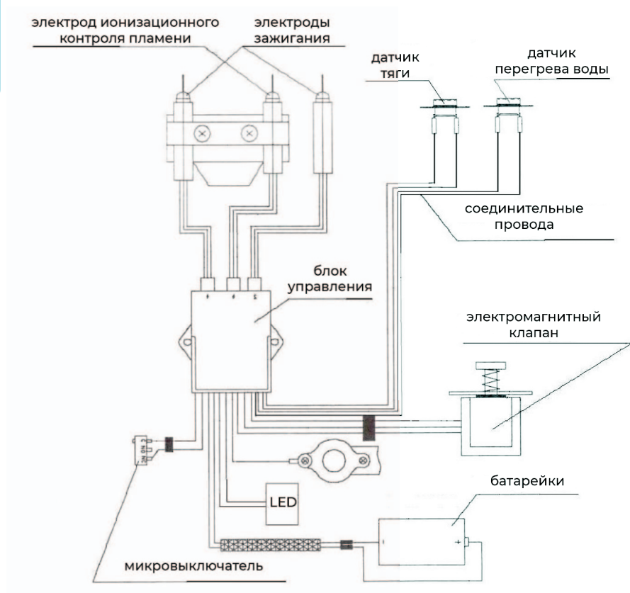
Рис.2. Схема электрическая
